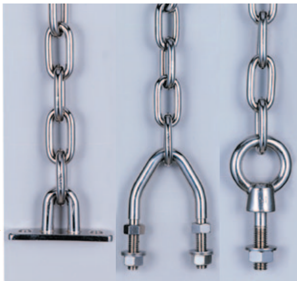
受け金具
